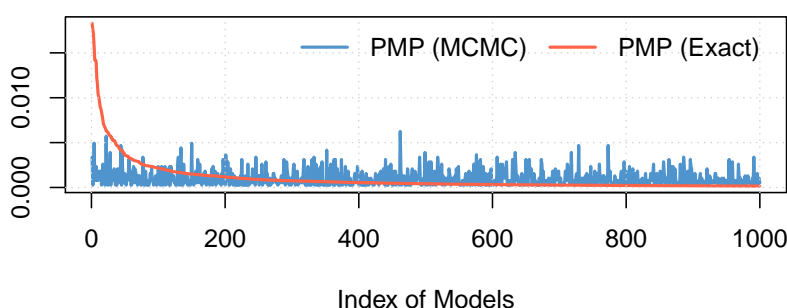
Posterior Model Probabilities (Corr: 0.1172)
