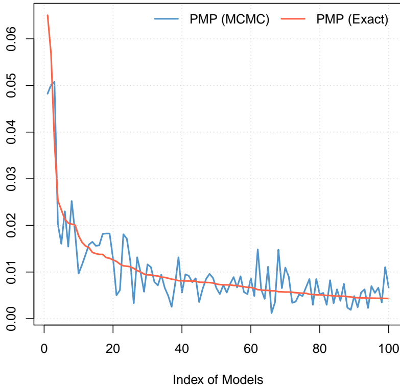
Posterior Model Probabilities (Corr: 0.8976)
