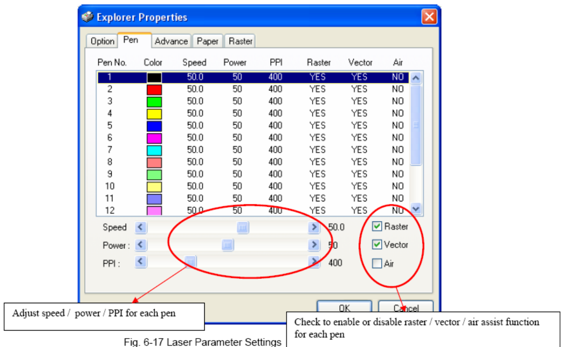
Fig. 6-17 Laser Parameter Settings
